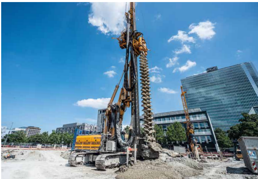
Baugrubenherstellung im Mixed-in-Place-Verfahren beim Projekt Parkstadt Schwabing in München
